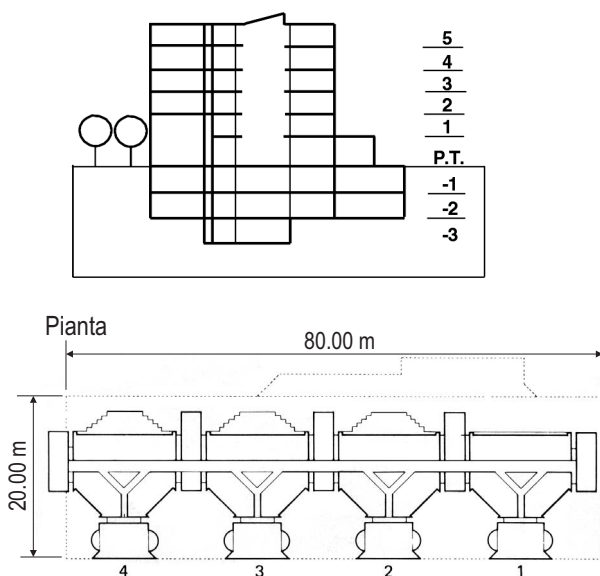
Sezione tipo
